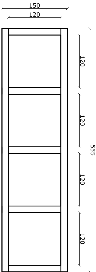
WIDOK FRONT
